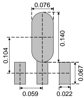
SOT-89
