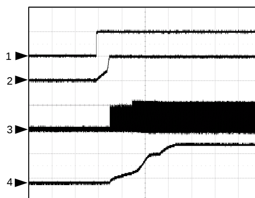
Enable, Hot Plug-In PWM, ENA=H
