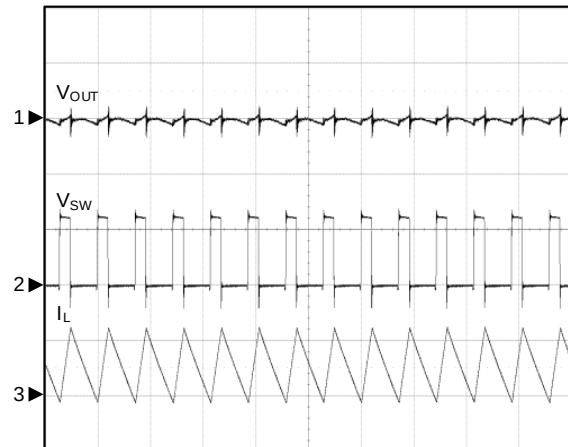
Vout Ripple
