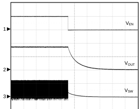
Shutsown
