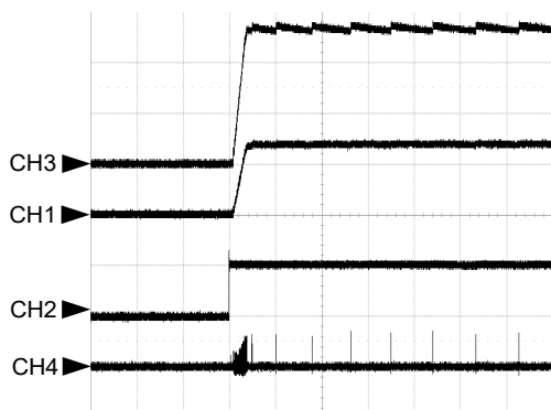
Enable VCC - No Load
