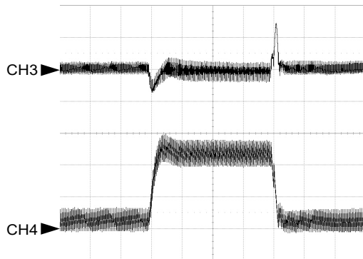
Load Transient-Load=1.2A<-->12A
